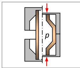
Slika 2.1. Oblikovanje cijevi
